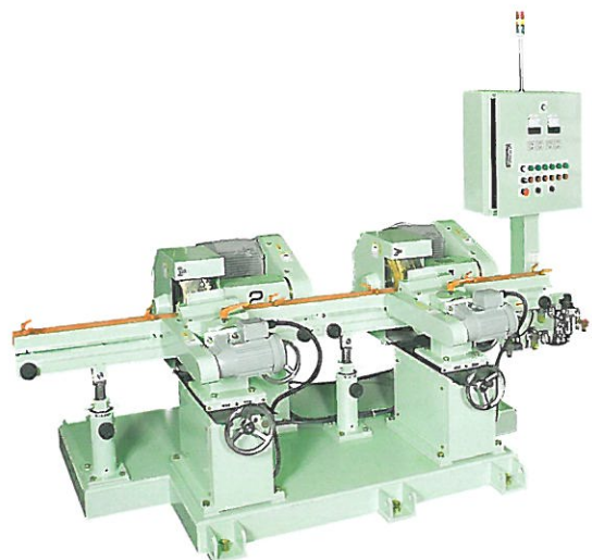
2連型 NCB-50II-2H Twin type
