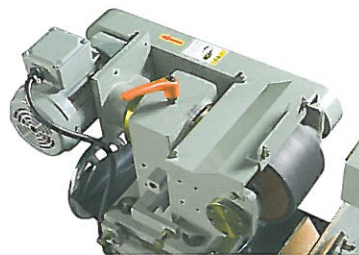
送り車部 Feed roller
